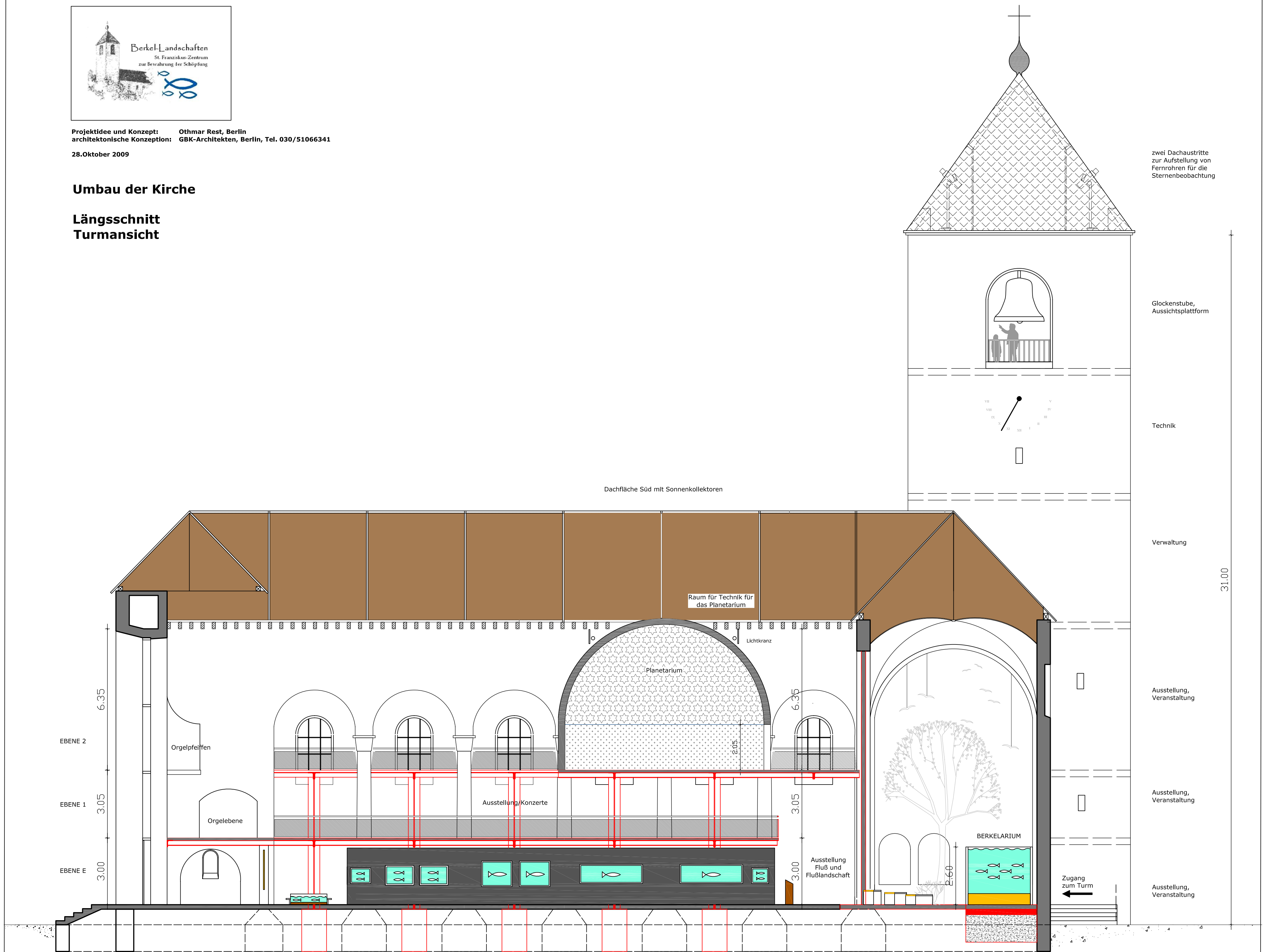
LÄNGSSCHNITT M 1:100
